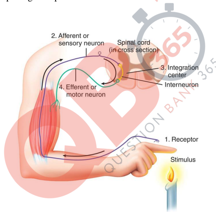
Fig. 7. Reflex arc
